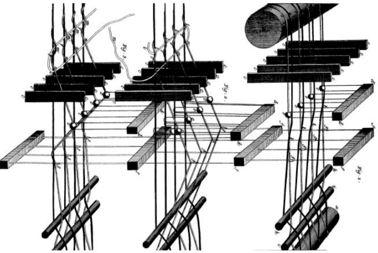
Garnier, Fonctions des Traverses du Mécanisme à Coton.
