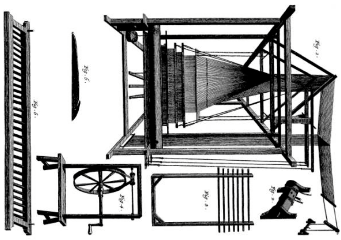
Gazier, Mètier à Gaze vu en face.
