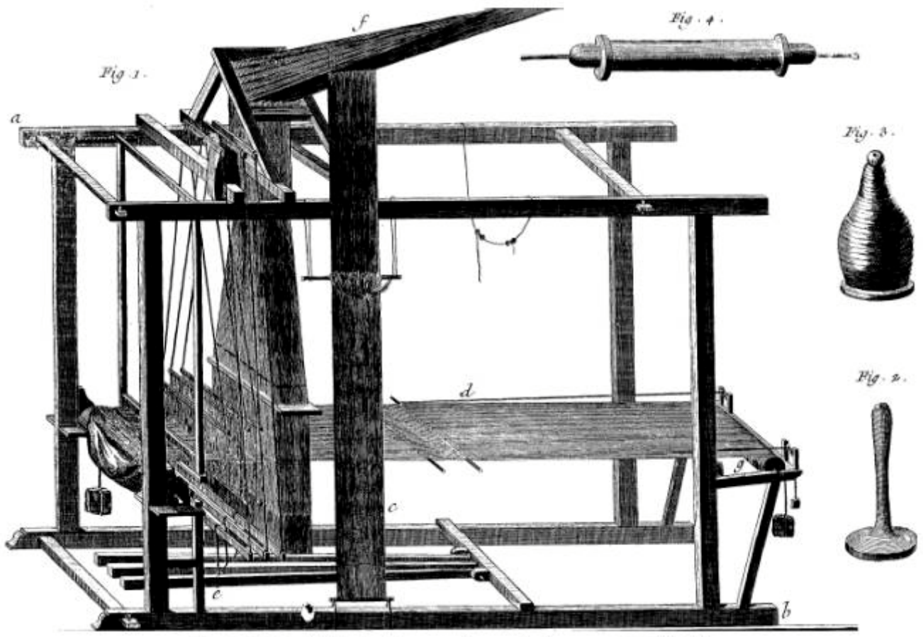
Gazier, Mètier à Gaze vu sur la longueur et Détails.
